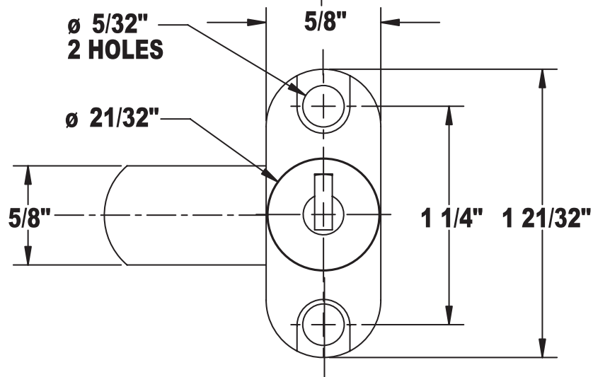
90° ROTATION CB-194
